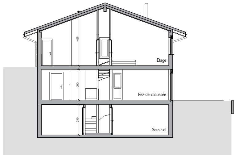
Coupe
